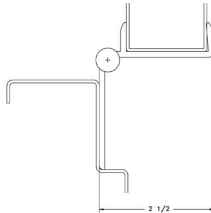
DOOR OPEN 90°
